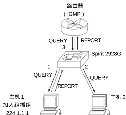
图 8-1 主机 1 加入组播组
