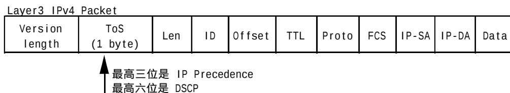
图 12-2 IP Precedence 和 DiffServ 的优先级位
