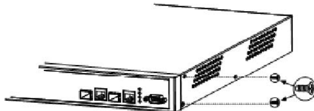
图 2-2 从交换机上拧下螺丝
