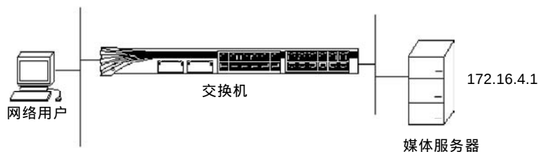
图 7-5 二层静态组播配置示例
