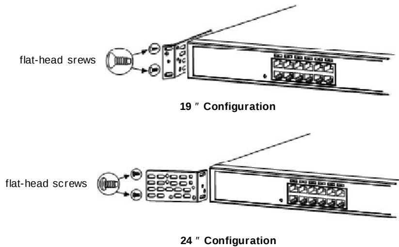
图 2-3 将法兰安装在交换机前部
