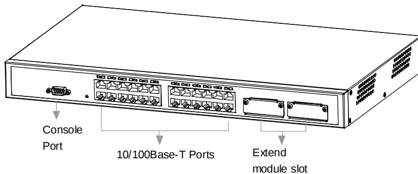
图 1-1 联想天工 iSpirit 2928G 交换机模型
