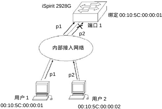
图 10-1 用户从绑定的端口接入网络
