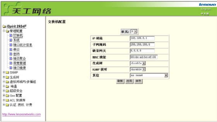
图 16-9 管理配置页面
