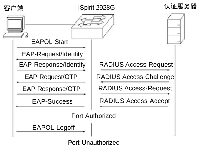
图 9-4 客户端发起认证的协议交互
