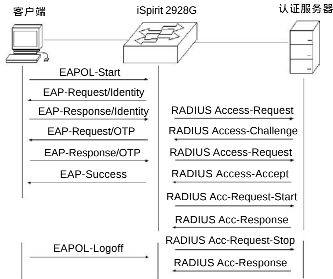
图 9-7 协议流交互
