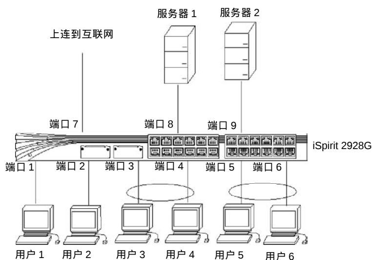
图 5-3 一个私有 VLAN 组
