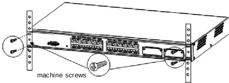
图 2-5 将交换机安装到机柜里
