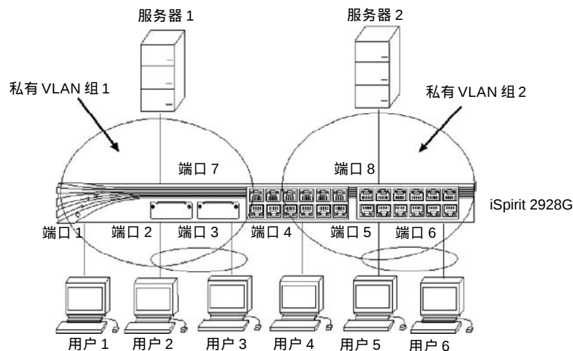
图 5-2 两个私有 VLAN 组
