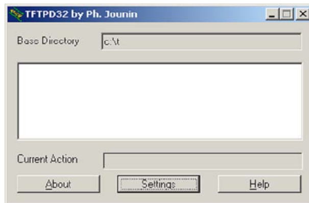
图 2-5 TFTPD32 界面图
