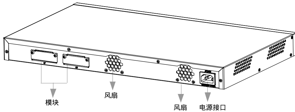
图 1-5 iSpirit 2928G 交换机后面板
