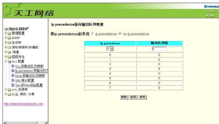
图 16-34 ip precedence 值到输出队列映射配置页面
