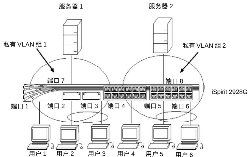
图 5-4 两个私有 VLAN 组
