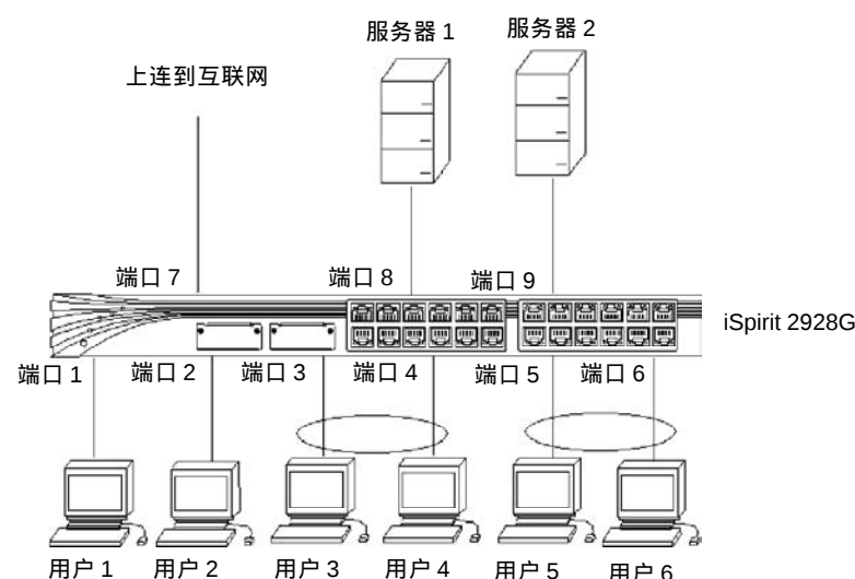
图 5-1 一个私有 VLAN 组
