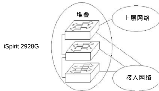
图 11-1 菊花链方式的堆叠
